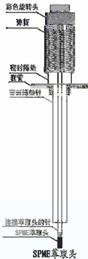
固相微萃取(SPME)萃取器
